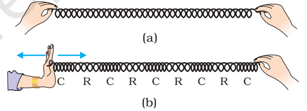
चित्र 11.5: स्लिंकी में अनुदैर्घ्य तरंग
