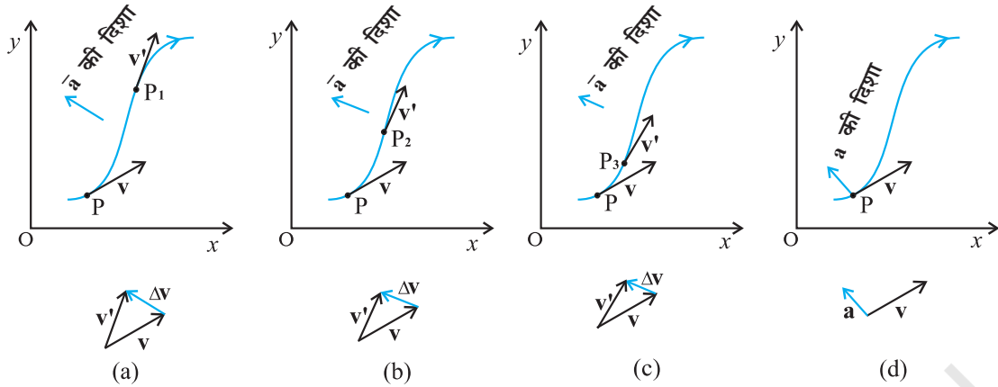
चित्र 3.15 तीन समय अंतरालों (a) \Delta t_1 , (b) \Delta t_2 , (c) \Delta t_3 ( \Delta t_1 > \Delta t_2 > \Delta t_3 ) के लिए औसत त्वरण \bar{a} (d) \Delta t \rightarrow 0 सीमा के अंतर्गत औसत त्वरण वस्तु के त्वरण के बराबर होता है।
